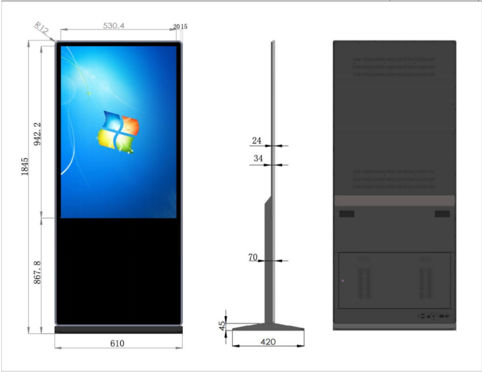
43寸落地红外广告机
